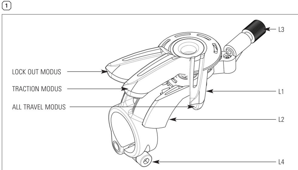
Fernbedienungshebel
