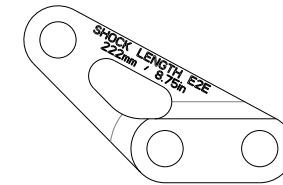
SHOCKMOUNT 222
