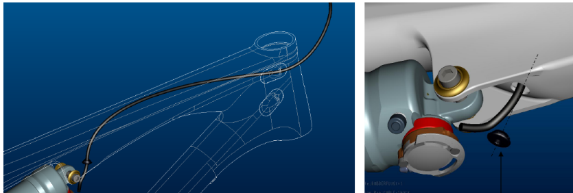
Schieben sie den Gummiring auf die Kabelhülle
